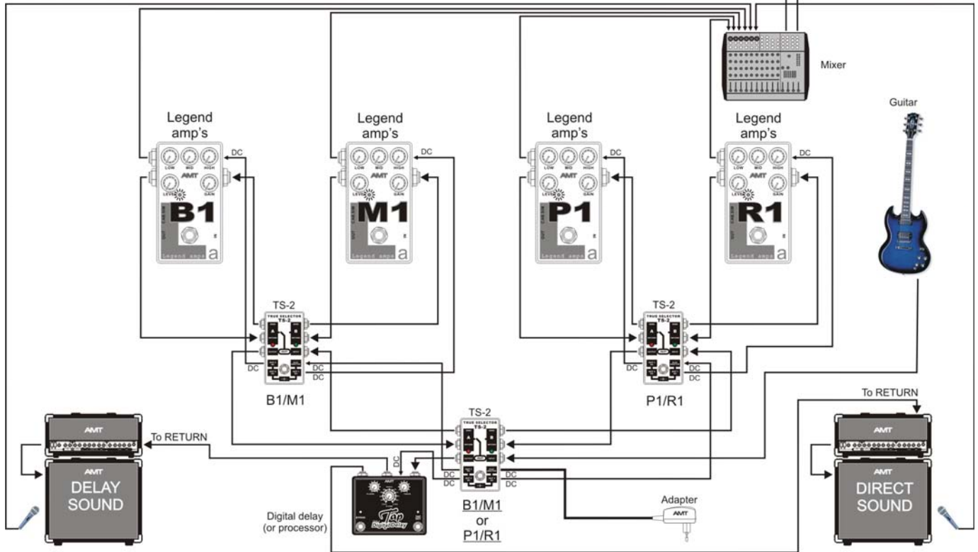
Legend-P1 Block-diagram. Legend-P1 Блок-схема.
